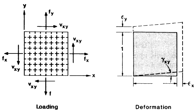
Fig. 2 — Membrane element
